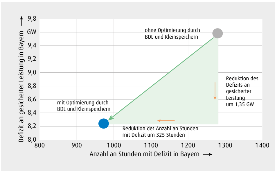
Bild 3. Reduktion des Defizits an gesicherter Leistung und der Anzahl an Stunden mit Defizit durch optimierten Einsatz von bidirektionalem Laden (BDL) und Kleinspeicher
